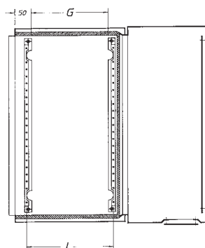
section Y - Y with open door
