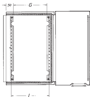
section Y - Y with open door
